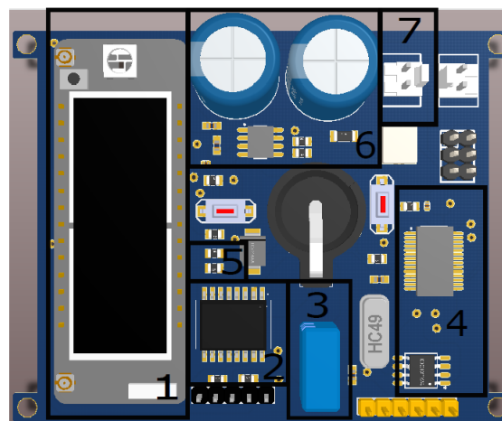
Figura 7. Prototipo de registrador de monitoreo de intensidad de lluvia.
