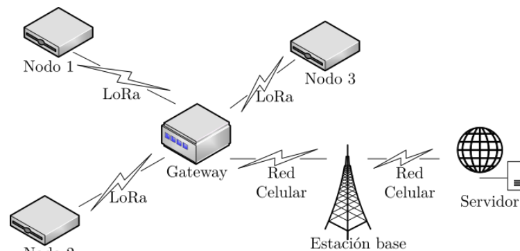
Figura 3. Esquema general de transmisión de datos basado en la tecnología LoRa.
