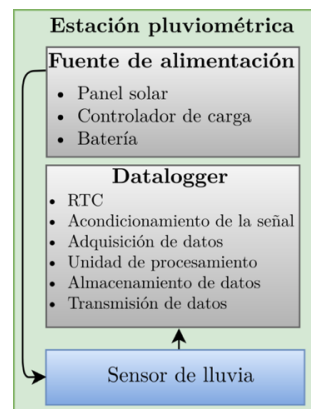
Figura 6. Estructura general de una estación pluviométrica con sensor de intensidad de lluvia.
