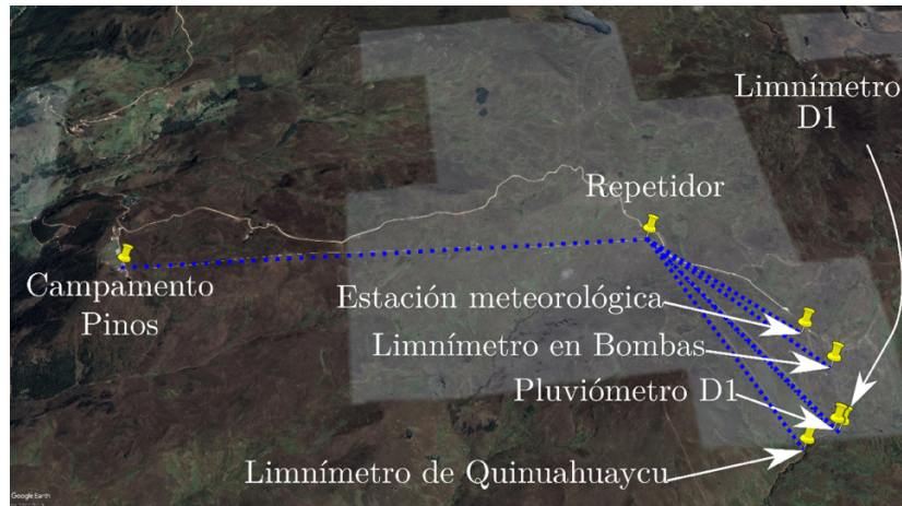
Figura 4. Topología de la red inalámbrica de sensores basada en la tecnología LoRa.
