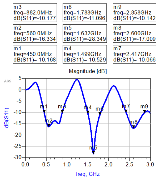
Figura 4. Parámetro S11 de la antena fractal alfombra de Sierpinski con alimentación en el puerto 2.
