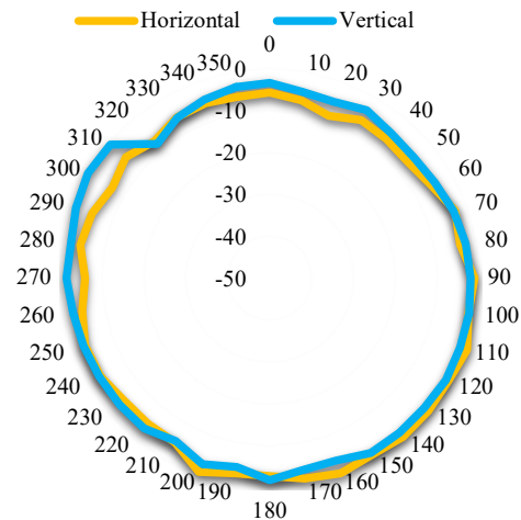
Figura 12. Diagrama normalizado de radiación en el plano horizontal y vertical para la antena AFPA4.
