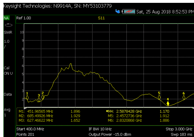
Figura 10. Mediciones del VSWR de la antena fractal alfombra de Sierpinski con puerto de alimentación 2.
