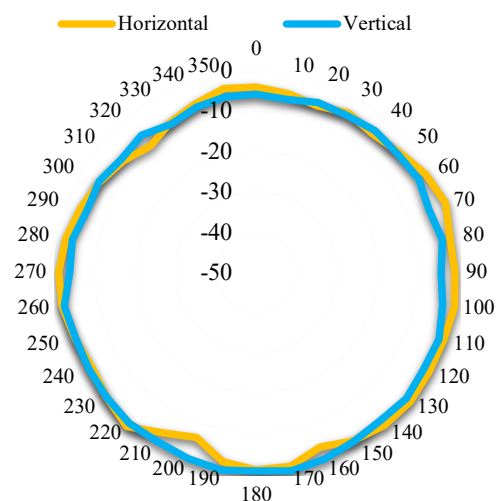
Figura 13. Diagrama normalizado de radiación en el plano horizontal y vertical para la antena AFPA2.
