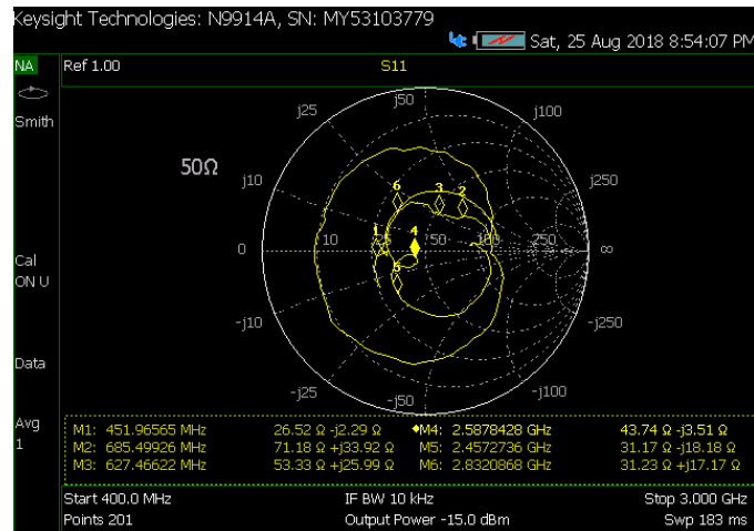
Figura 11. Mediciones de la impedancia de entrada de la antena fractal alfombra de Sierpinski con puerto de alimentación 2.
