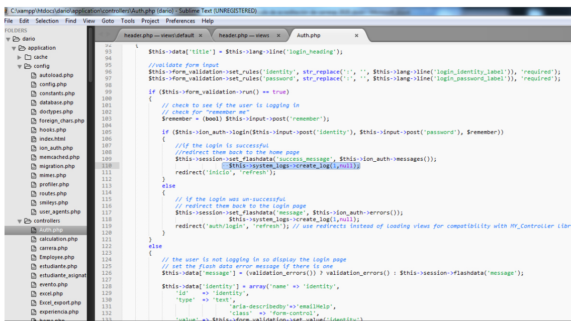
Figura 8. Fragmento de código del registrar usuario donde se aplica la librería System_logs .
