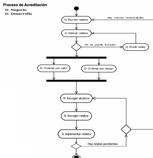
Figura 10. Diagrama de iteración de los casos de pruebas de aceptación.
