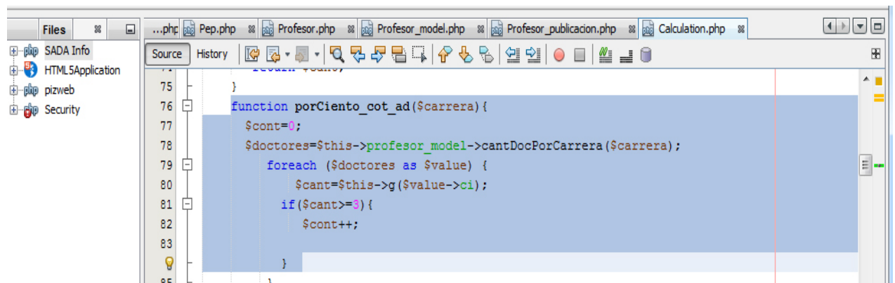
Figura 9. Fragmento de código del proyecto SADA Info.
