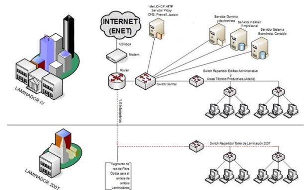
Figura 2 Diagrama de la configuración de red anterior
