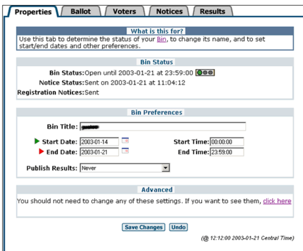
Figura 3 Configuración de una elección en BallotBin.
