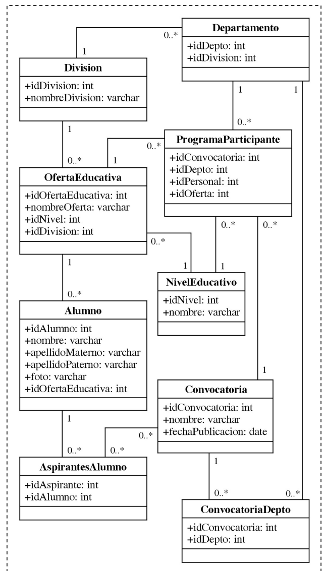
Figura 7 Diagrama de clases del sistema.
