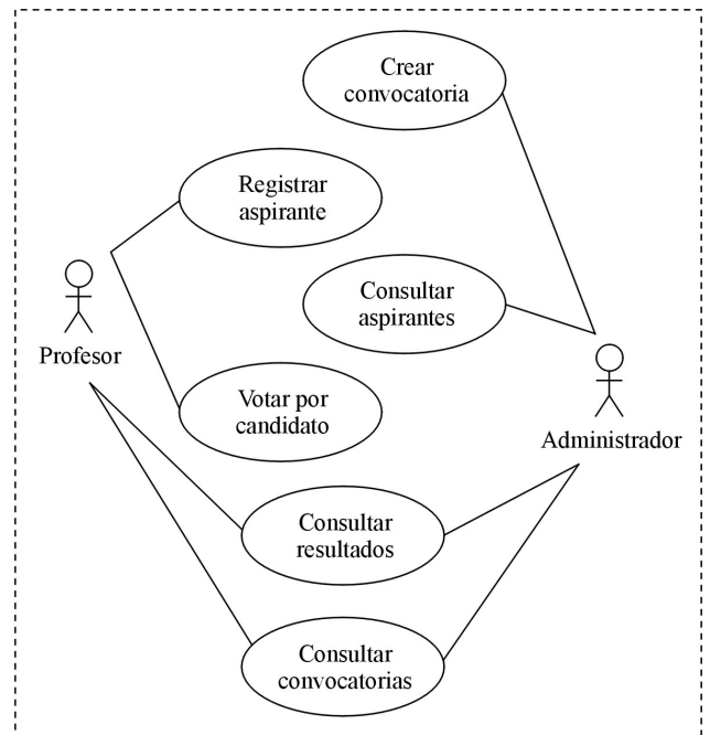
Figura 6 Diagrama de casos de uso.
