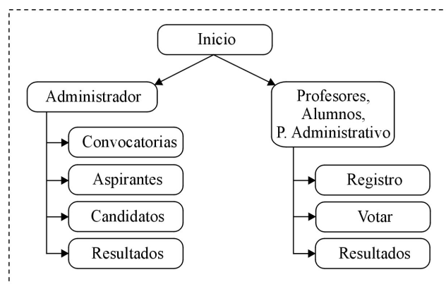
Figura 9 Mapa de navegación del sistema.
