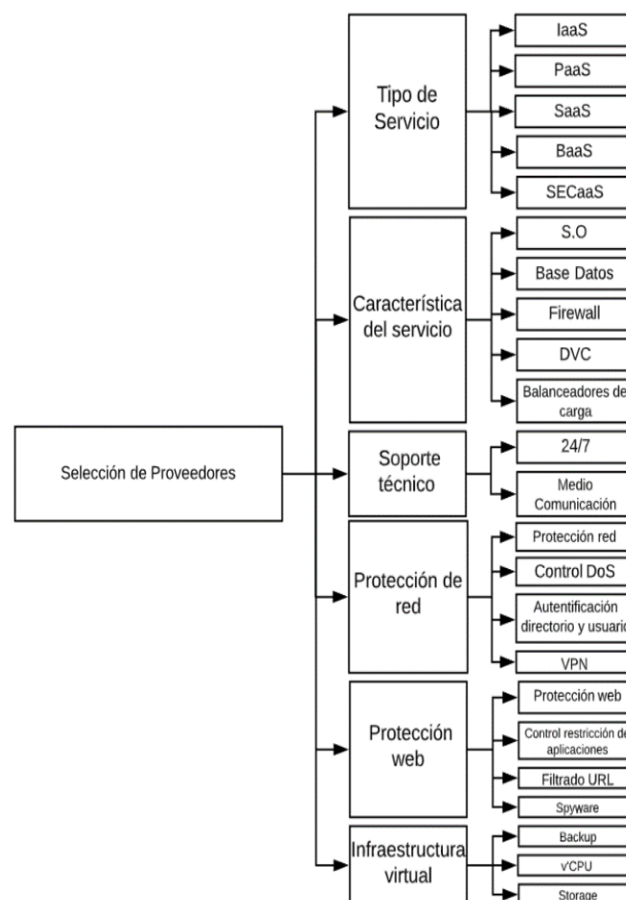
Figura 2 .Modelo jerárquico de selección de proveedores.
