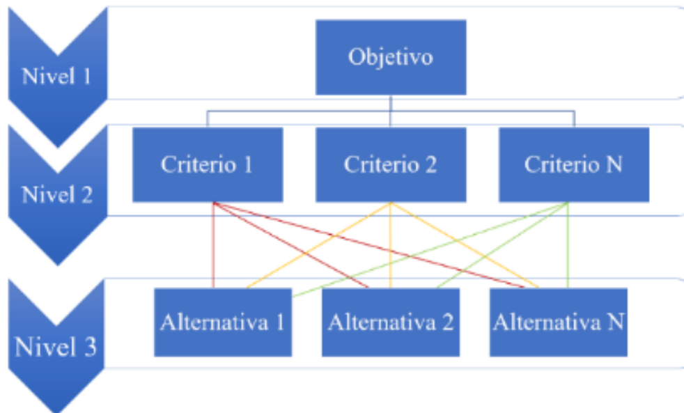
Figura 1. Estructura general del modelo AHP.
